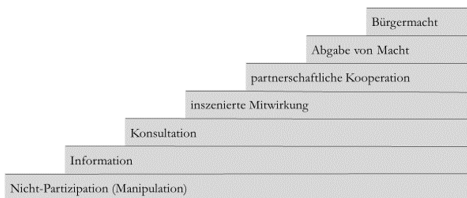
Abbildung 1: Beteiligungsleiter
